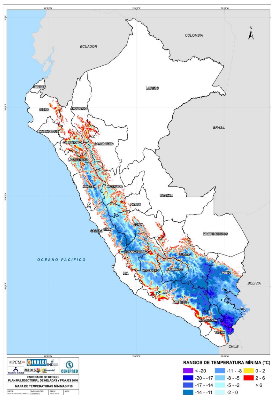
Figura N° 1: Mapa de Temperaturas mínimas del percentil 10 – Mes de Julio
